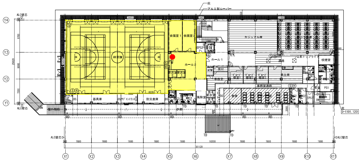
2階平面図
